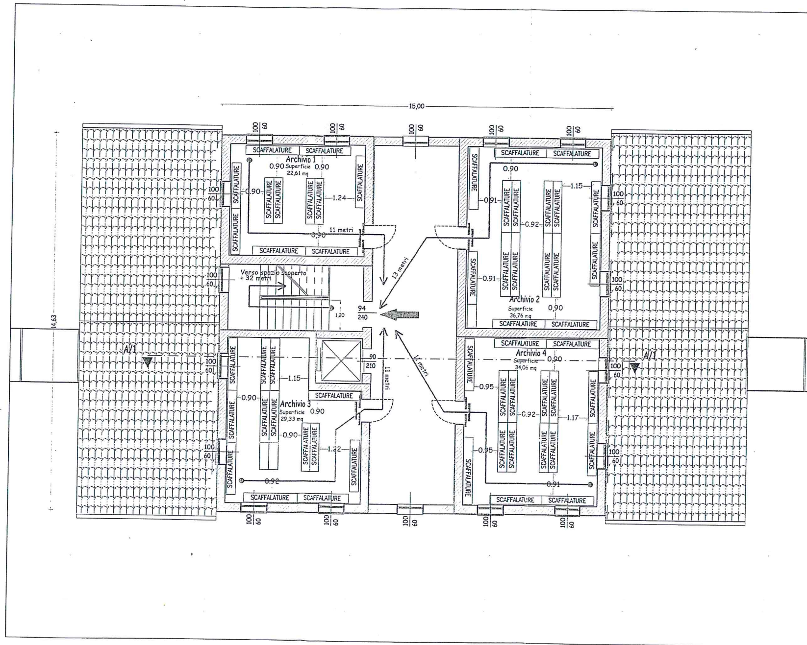
PIANTA PIANO SOTTOTETTO - SCHEMA INDICAZIONE SCAFFALI E VIE DI ESODO Scala 1:100
