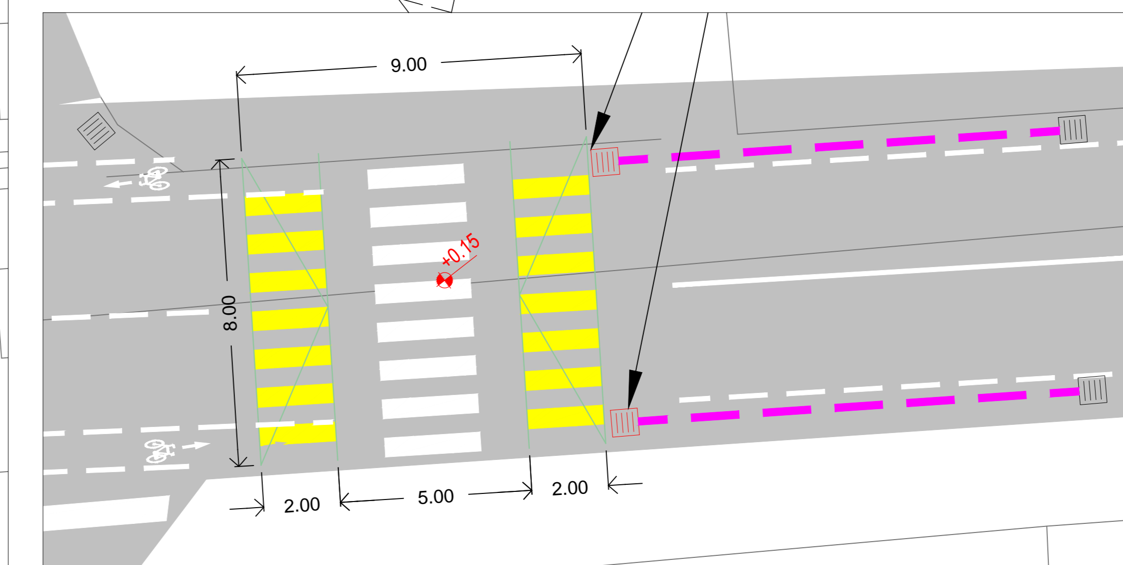
PARTICOLARE ATTRAVERSAMENTO RIALZATO SCALA 1:100
