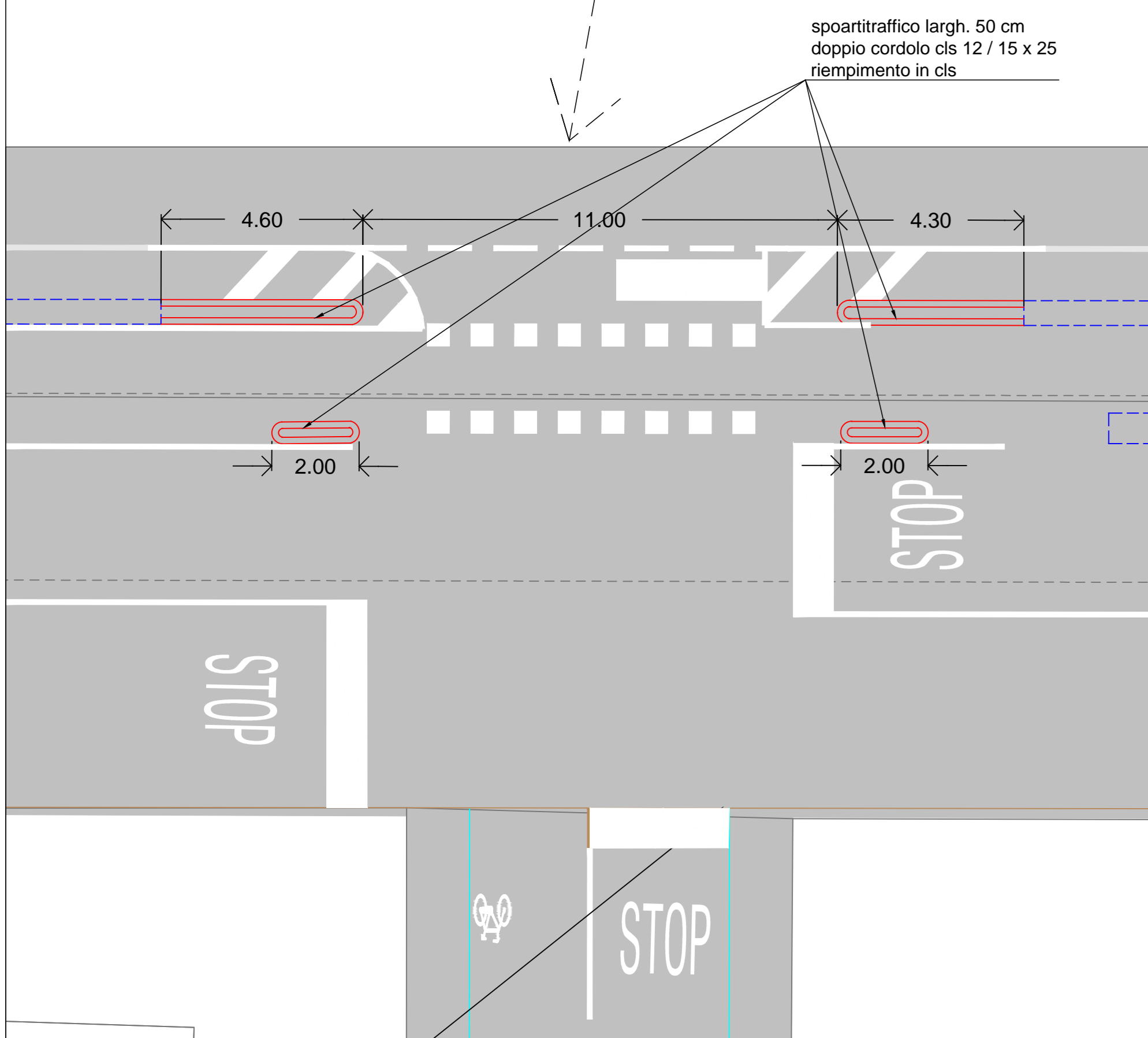
PARTICOLARE INTERSEZIONE SP 420 - VIA MANTEGNA SCALA 1:100
