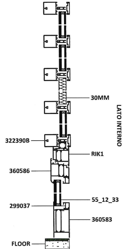
SEZIONE BB
